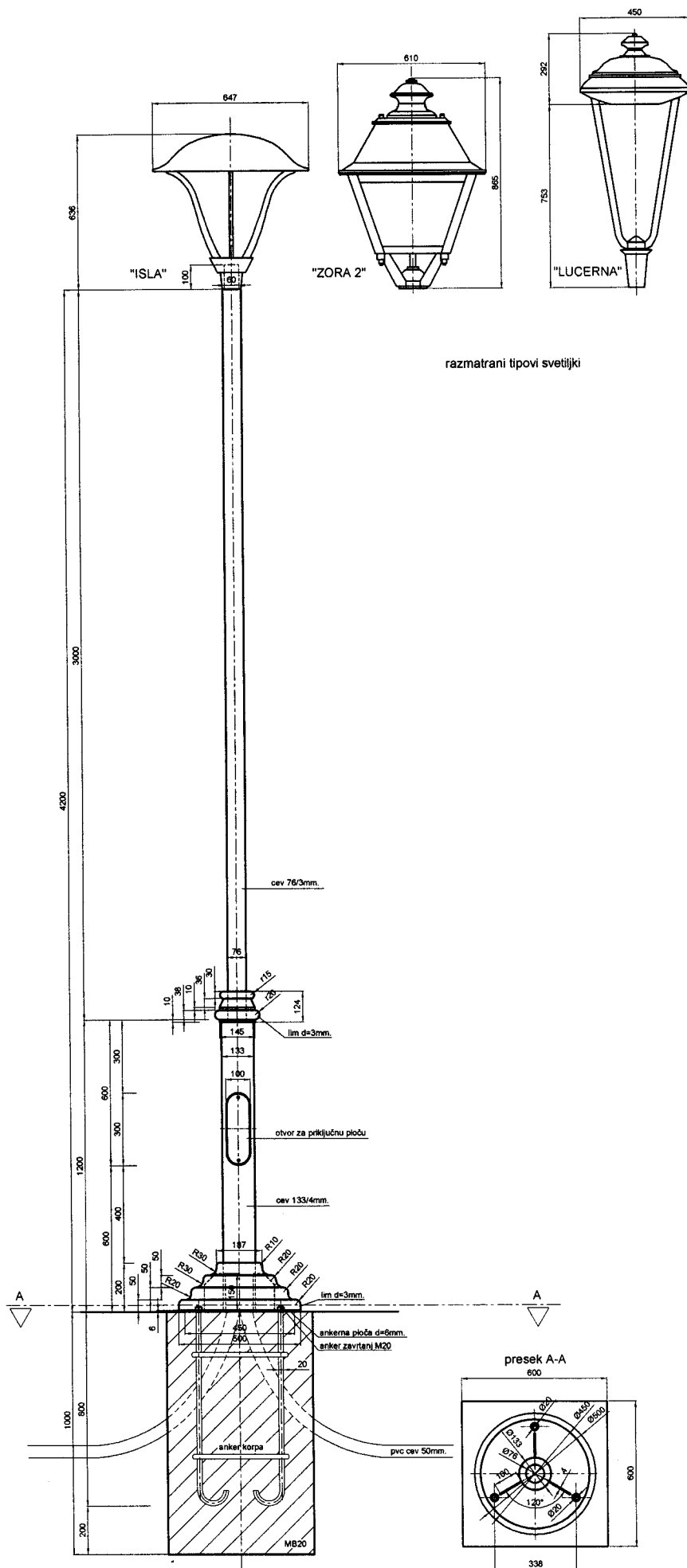
DS.1 Detalj stuba i temelja
